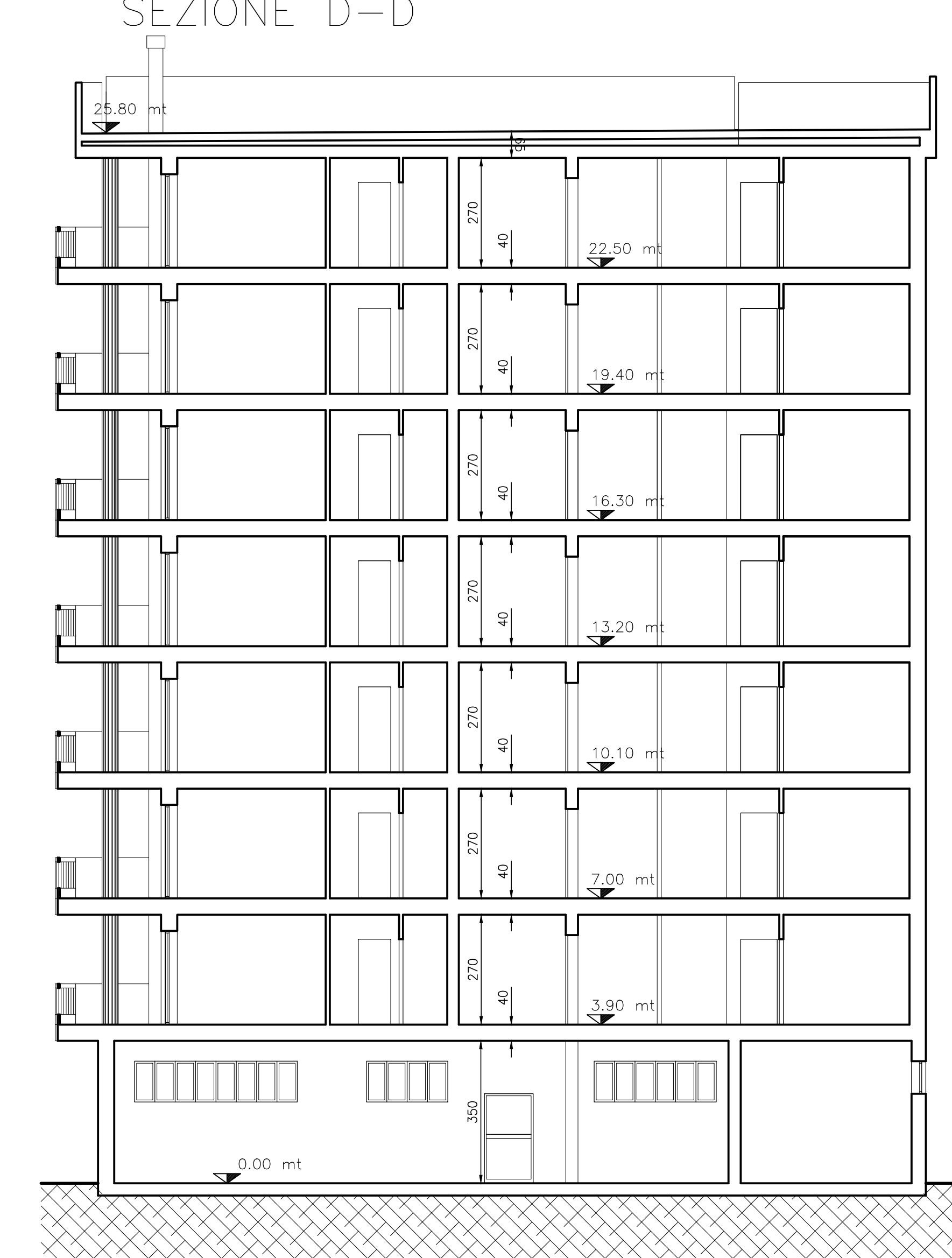
SEZIONE D-D
