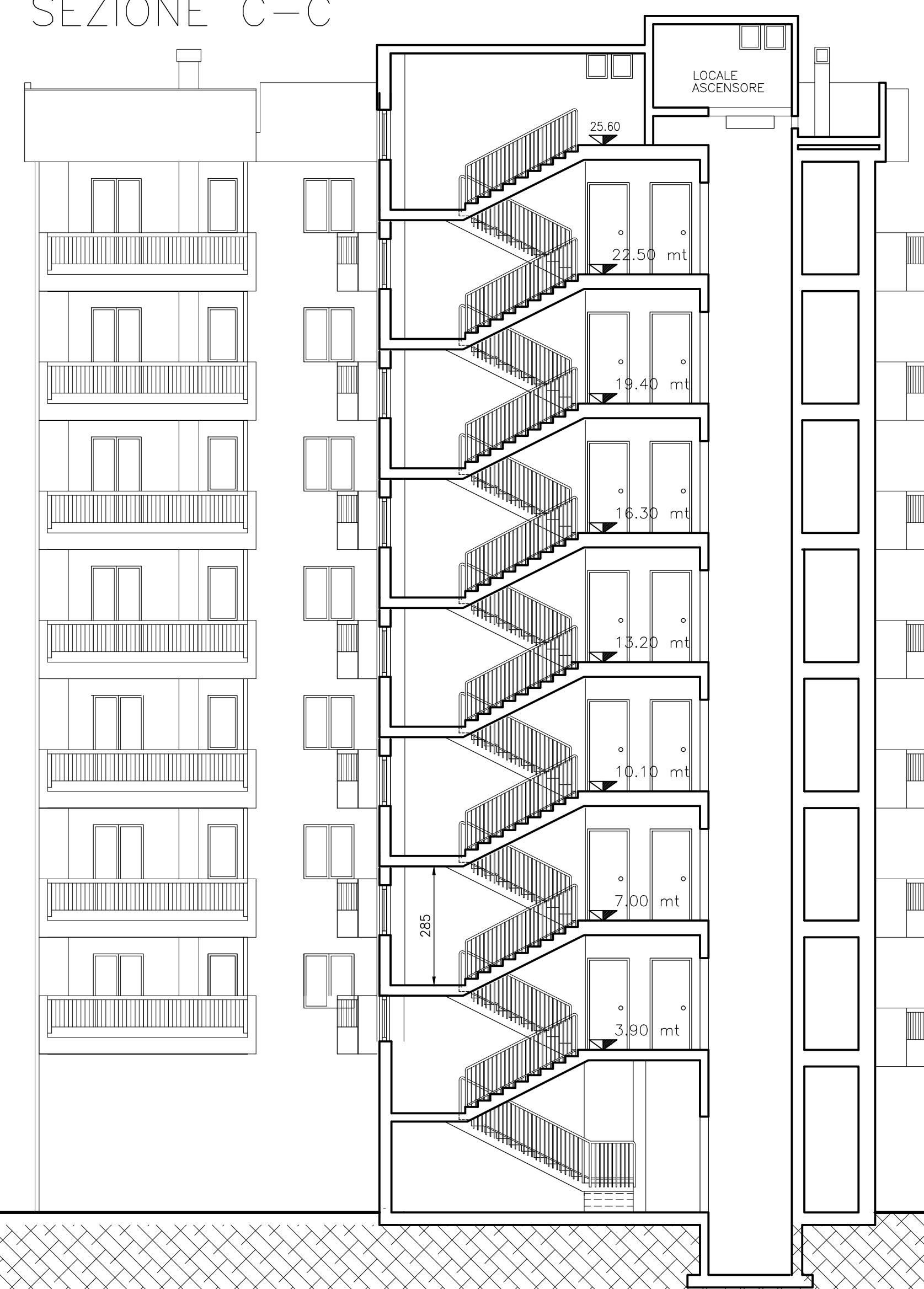
SEZIONE C-C
