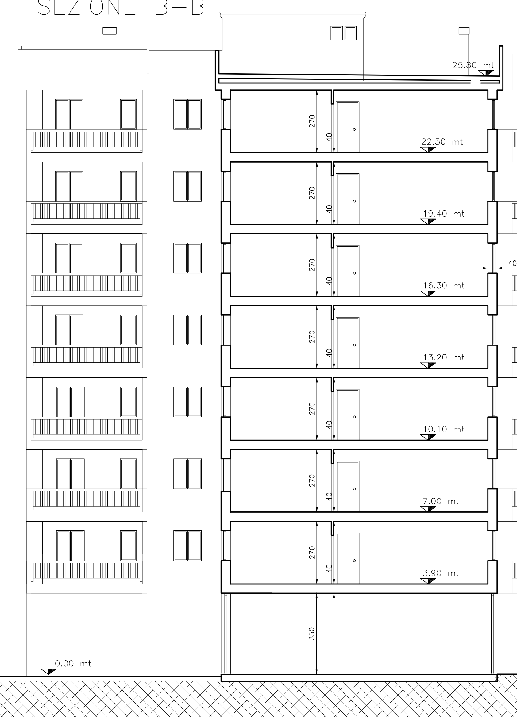
SEZIONE B-B
