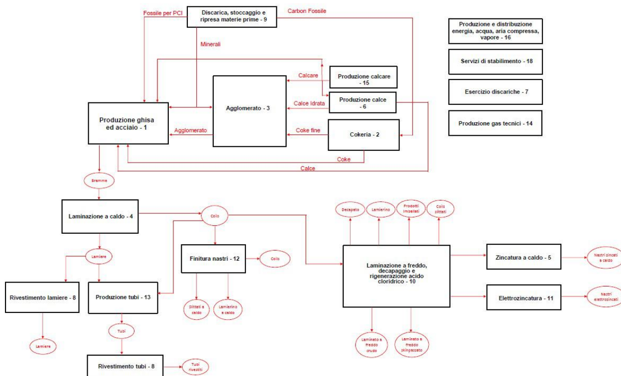
Schema di flusso del processo produttivo dello stabilimento siderurgico di Taranto
